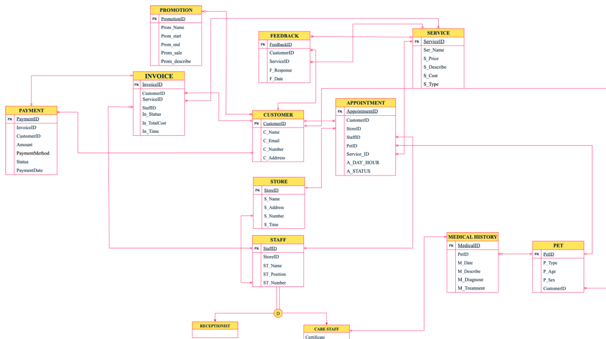
Hình 2.1. Sơ đồ mô tả mối quan hệ thực thể ER (hoặc ERR) của PetCare
