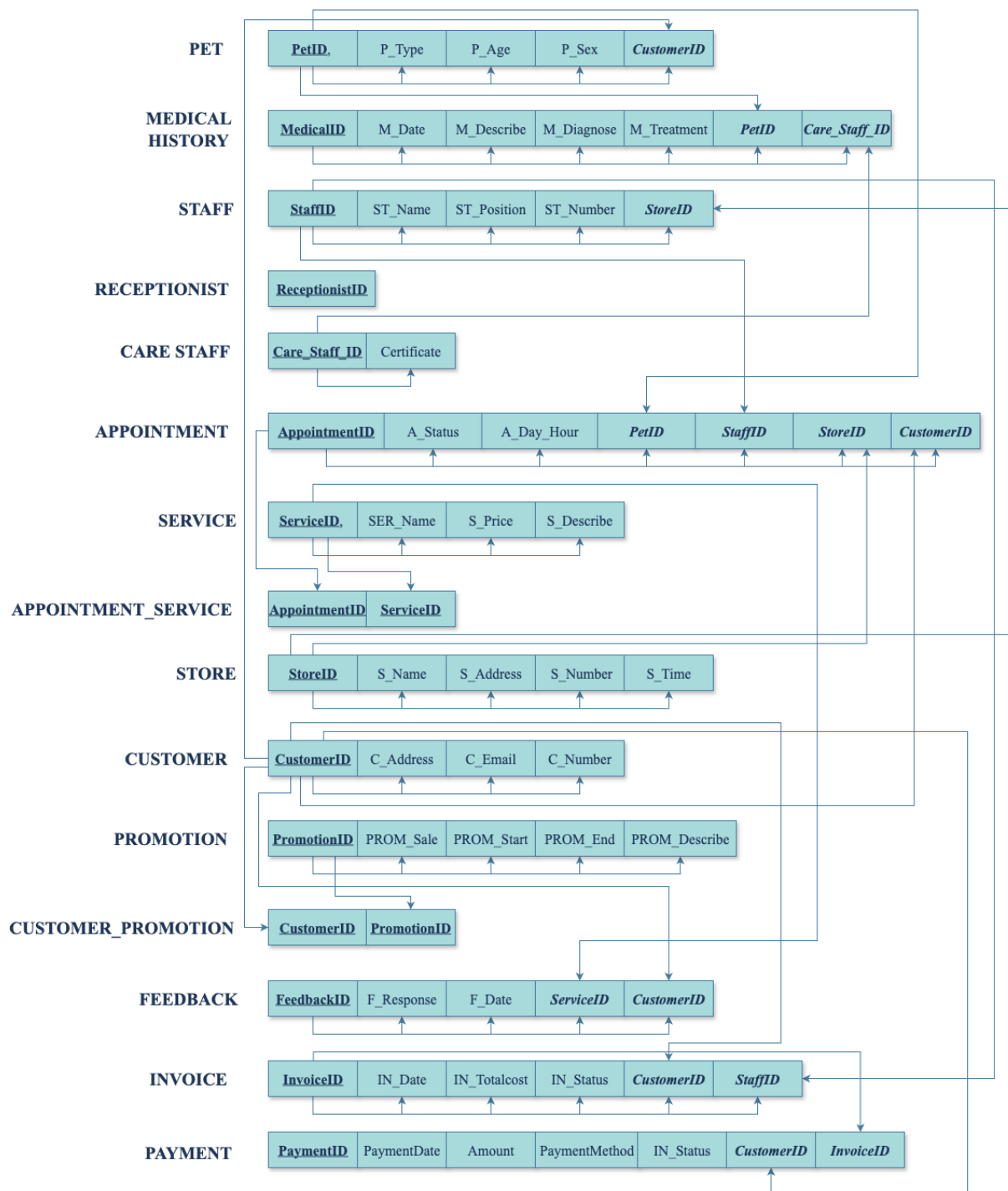
Hình 3.1. Sơ đồ các phụ thuộc hàm của các quan hệ
